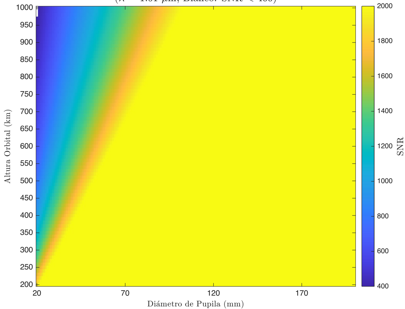
SNR - Refractivo - Detector 2 ( \lambda = 1.61 \mu\text{m} , Blanco: SNR < 400)
